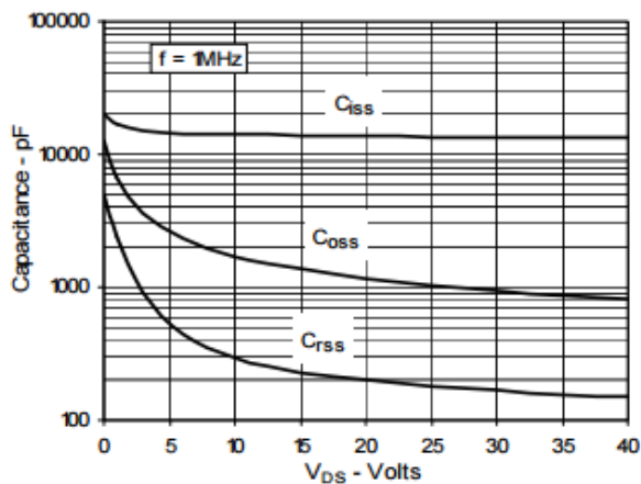
Fig. 11. Capacitance
